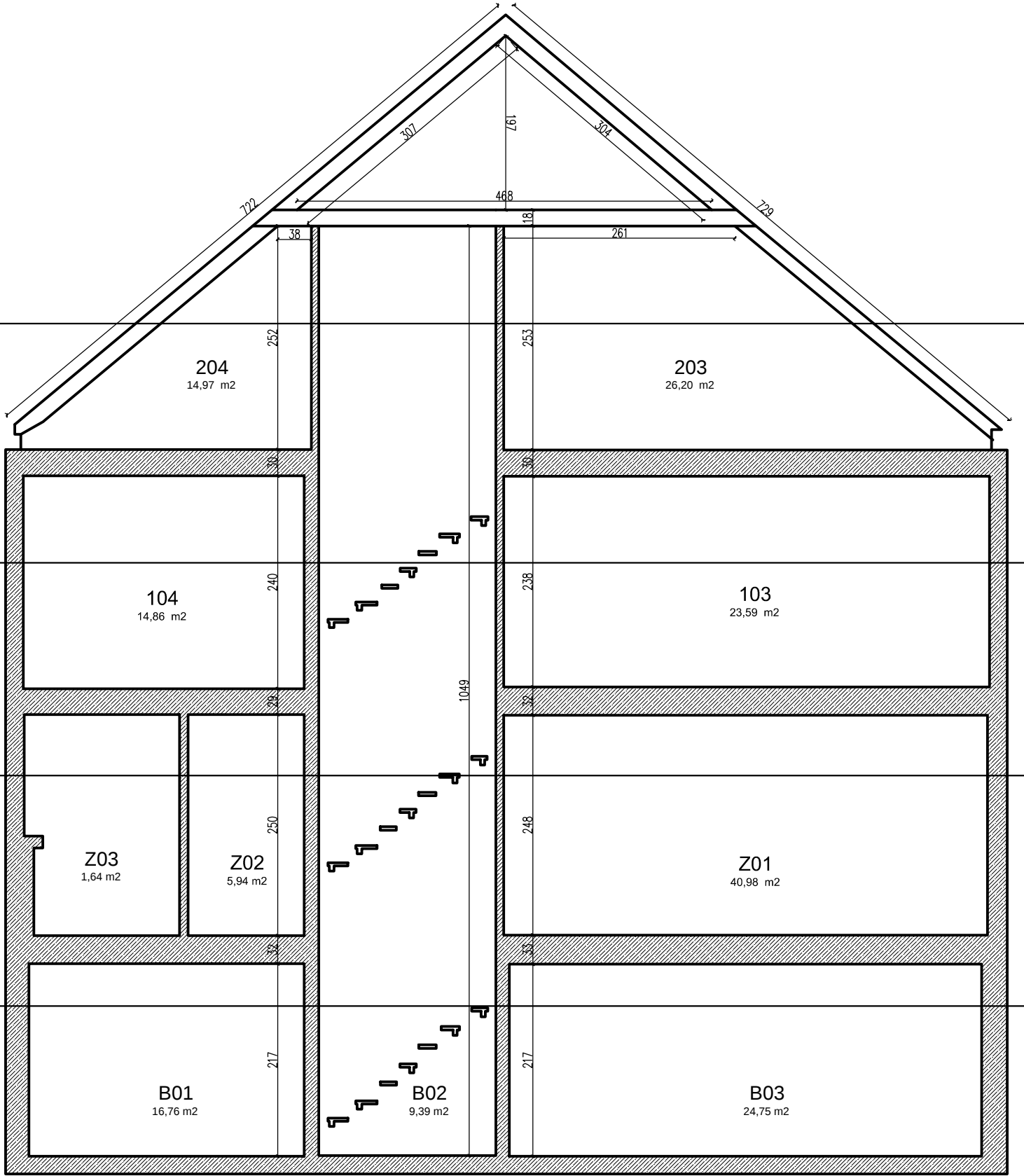
A-A KESİTİ
