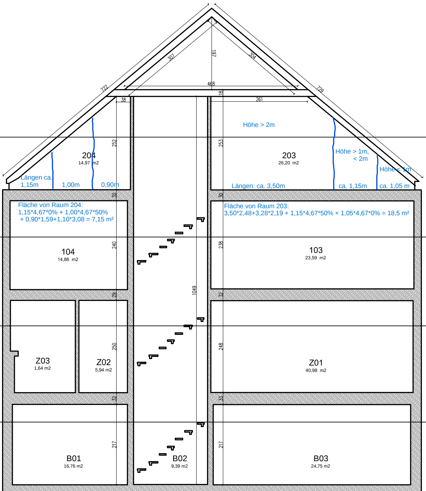
A-A KESİTİ
